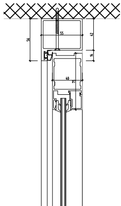
NovaOne Aluminiumrahmentürblatt raumhoch Vertikalschnitt
