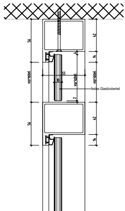
NovaOne Ganzglastürblatt mit Sturzprofil Vertikalschnitt
