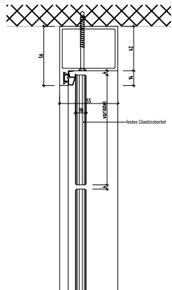
NovaOne Ganzglastürblatt mit Glasoblicht Vertikalschnitt
