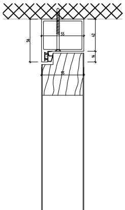
NovaOne 55 mm Volltürblatt raumhoch Vertikalschnitt
