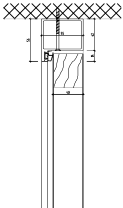
NovaOne 40 mm Volltürblatt raumhoch Vertikalschnitt
