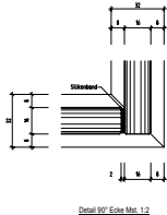
NovaOne 90° Ecke Horizontalschnitt
