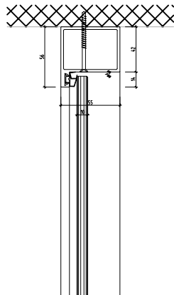
NovaOne Ganzglastürblatt raumhoch Vertikalschnitt
