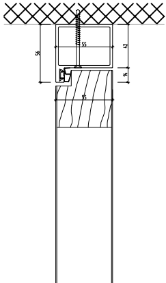
NovaOne 55 55 mm Volltürblatt raumhoch Vertikalschnitt
