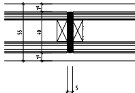
NovaOne 55 Glasstoss 5 mm mit schwarzer Kittfuge Horizontalschnitt
