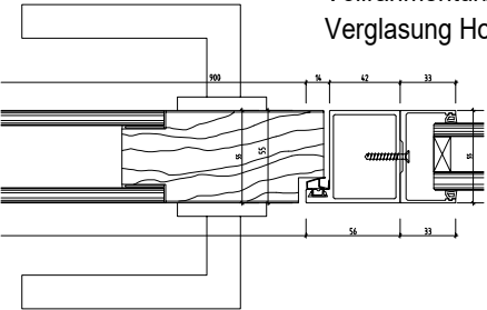
NovaOne 55 55 mm Volltürblatt Horizontalschnitt
