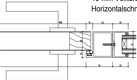
NovaOne 55 Aluminiumrahmentürblatt Horizontalschnitt
