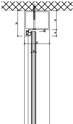
NovaOne 55 Ganzglastürblatt raumhoch Vertikalschnitt
