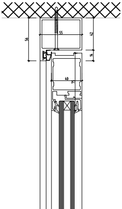
NovaOne 55 Aluminiumrahmentürblatt raumhoch Vertikalschnitt
