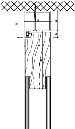
NovaOne 55 55 mm Vollrahmentürblatt mit 2-fach Verglasung Vertikalschnitt
