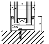
NovaOne 55 Bodenanschluss Vertikalschnitt
