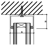
NovaOne 55 Deckenanschluss Vertikalschnitt
