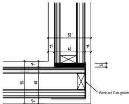
NovaOne 55 90° Ecke Horizontalschnitt
