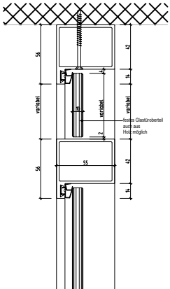
NovaOne 55 Ganzglastürblatt mit Sturzprofil Vertikalschnitt
