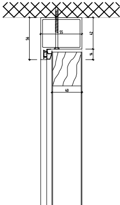
NovaOne 55 40 mm Volltürblatt raumhoch Vertikalschnitt
