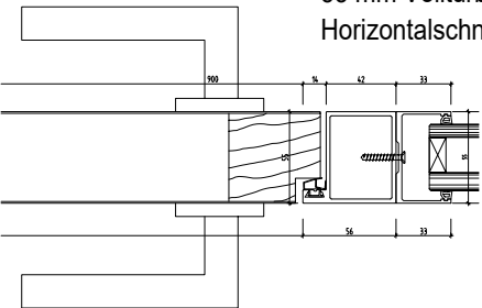
NovaOne 55 40 mm Volltürblatt Horizontalschnitt
