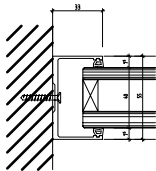
NovaOne 55 Wandanschluss Horizontalschnitt
